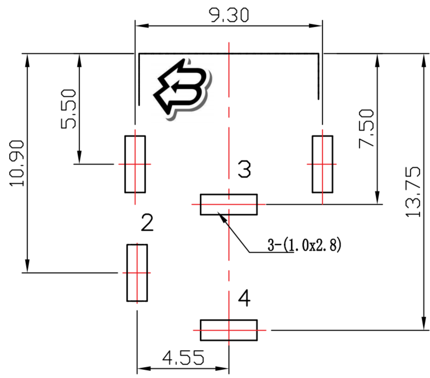
线路板开孔尺寸图
